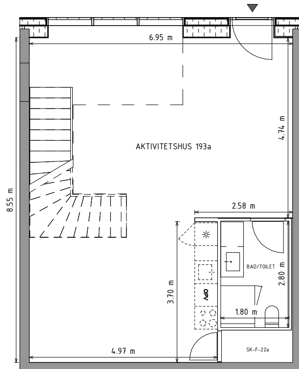
Etage 00
