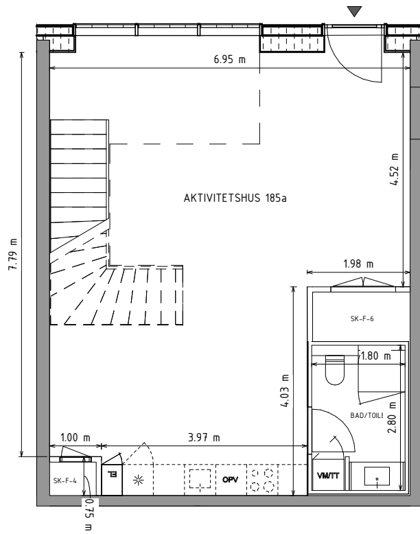
Etage 00
